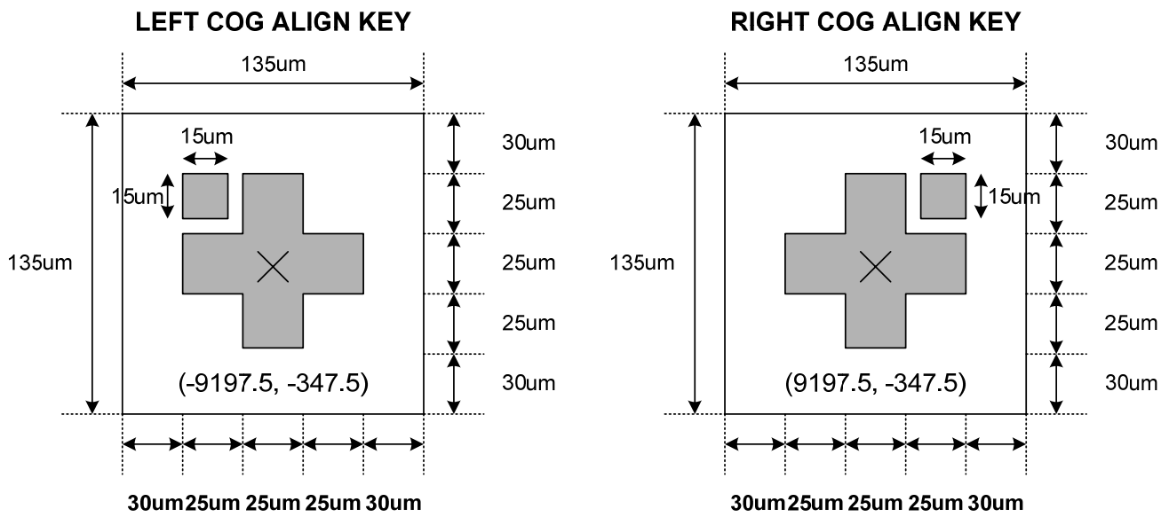
Fig 3. COG Align Keys
